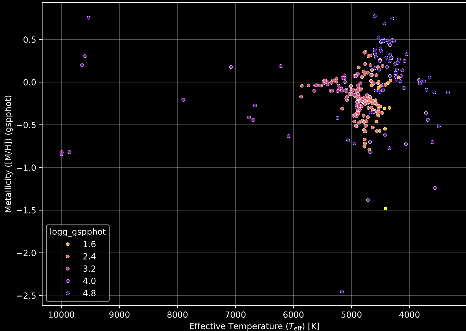
APOGEE DR17 Field: [160+24_btx] Stellar Population Parameters (n= 288)
